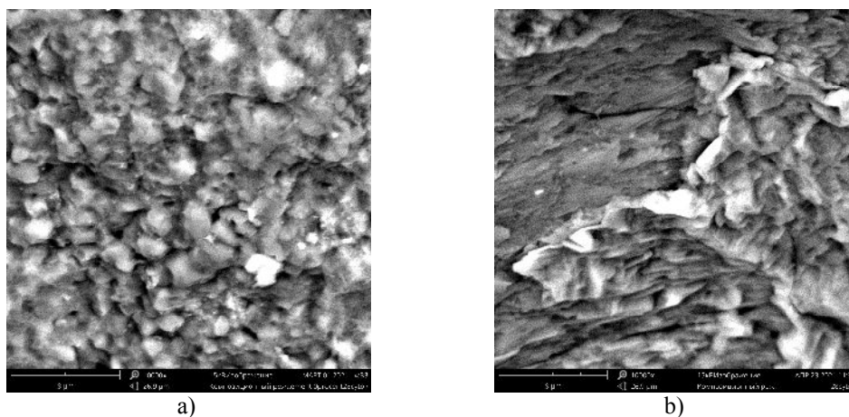
Рис. 8. Микроструктура контрольного цементно-песчаного камня (а) и модифицированного порошком WC (b) в возрасте 28 суток
