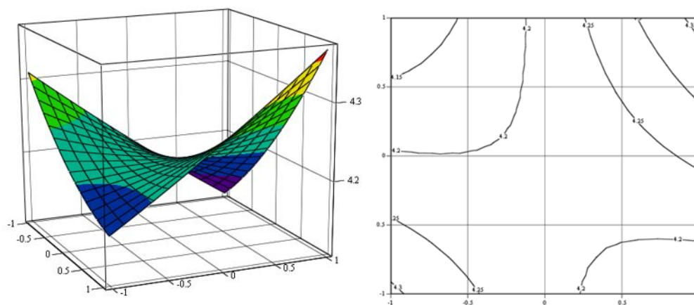
Рис. 2. Зависимость изменения прочности на растяжение при изгибе базальтофибробетона от процентного содержания фракций заполнителя (фр. 5–10/10–20) и процента фибрового армирования
